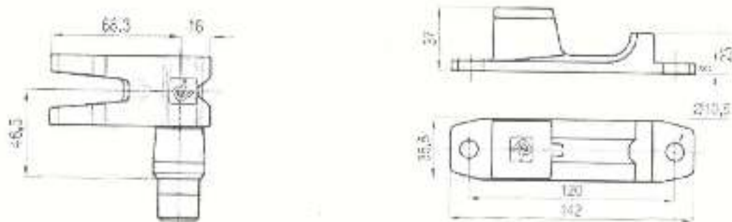
Рис. 2 – Присоединительные размеры кулачков запорных устройств.
